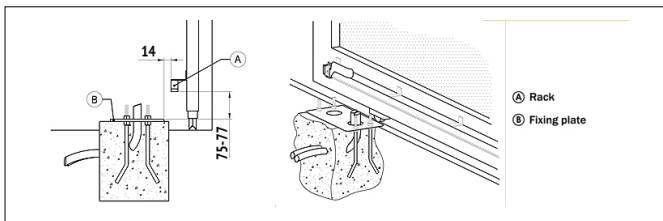
СТАНДАРТЕН НАЧИН НА МОНТАЖ
